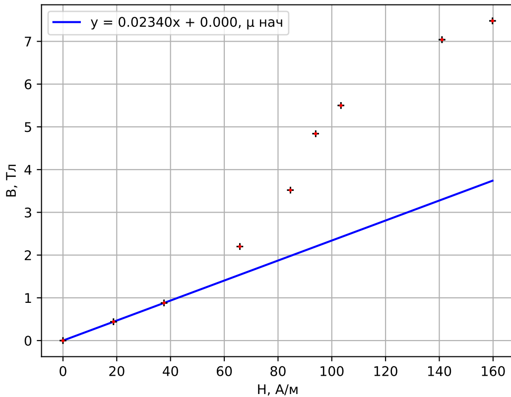
Зависимость В от Н, Fe-Ni
